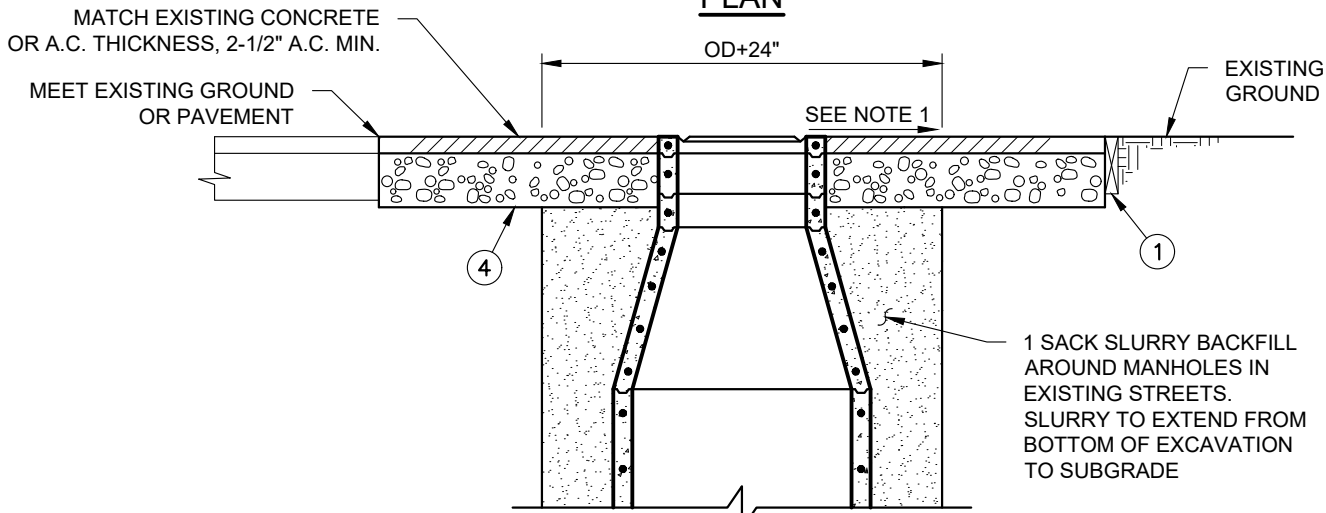
SECTION A-A
